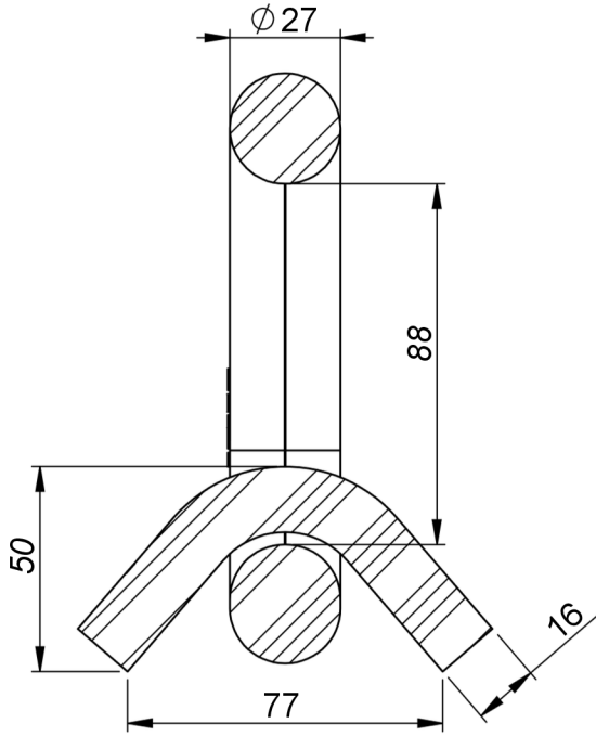
A-A
